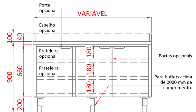
ELEVAÇÃO FRONTAL
