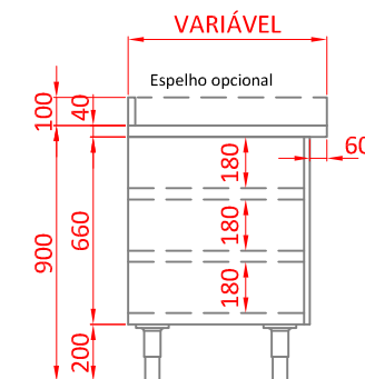
ELEVAÇÃO LATERAL
