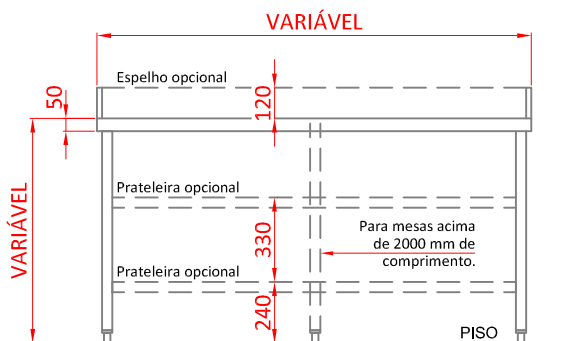
ELEVAÇÃO FRONTAL
