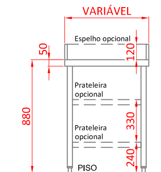
ELEVAÇÃO LATERAL
