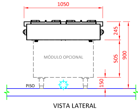
VISTA LATERAL
