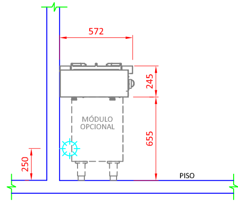
VISTA LATERAL
